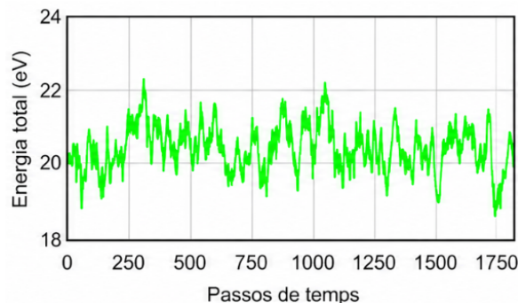
(b) Energia total en funció del temps.
