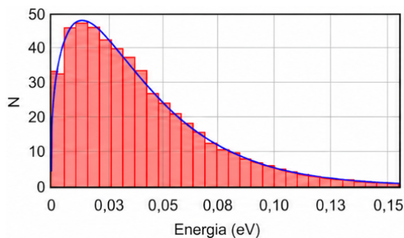
(a) Distribució d'energies.
